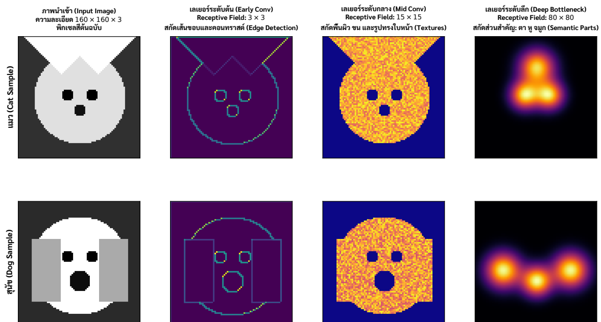
รูปที่ 5: การถอดรหัสพีเจเออร์ภายในโครงข่าย: วิวัฒนาการของ Receptive Field ตั้งแต่เลเยอร์ระดับต้น (ตรวจจับเส้นขอบ) ระดับกลาง (ตรวจจับลวดลายชน) จนถึงระดับลึก (ตรวจจับอวัยวะสำคัญบนใบหน้า)
